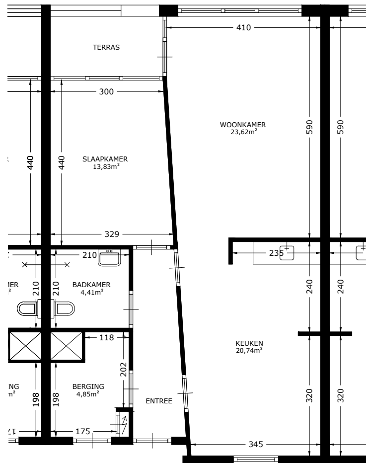
BEGANE GROND
