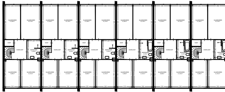
EERSTE VERDIEPING
